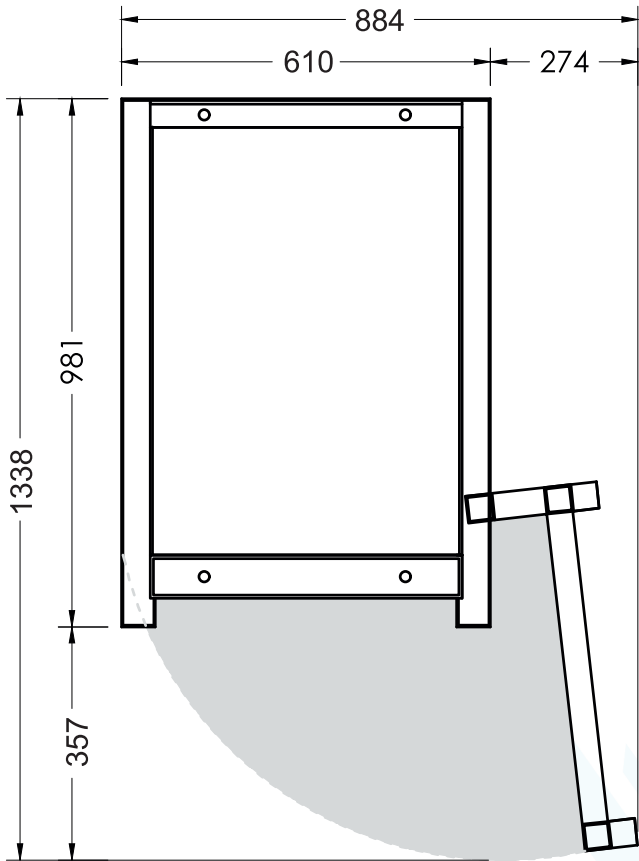
SECCIÓN HORIZONTAL
